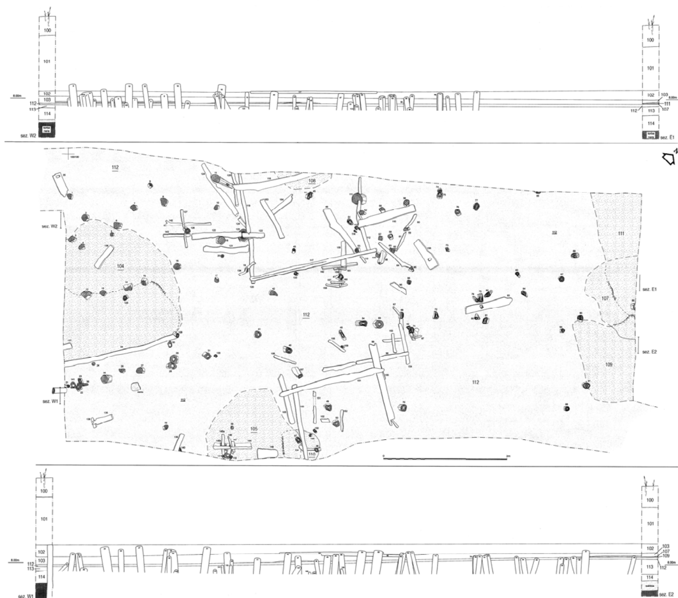
Fig.5. Tombola di Cerea. Pianta dello scavo del 1999 e sezioni W1-E2, W2-E1. Plan of excavated area in 1999 and W-E sections
